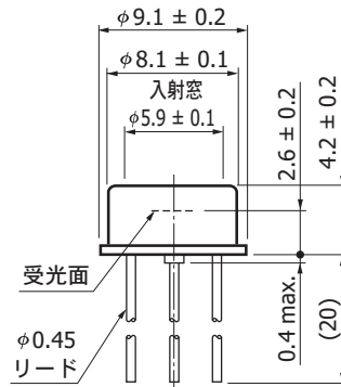
(2) S9251-10/-15
